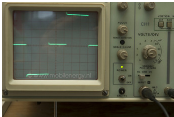
Foto: een gemodificeerde sinus in het echt
