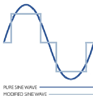
Plaatje: een zogenaamde gemodificeerde sinus
